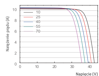
Krzywa prąd-napięcie JAM60S10-335/MR
